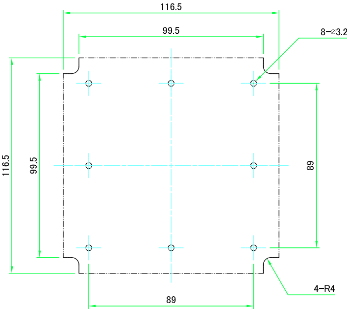
推奨基板形状 * 販売していません Recommended PCB dimension * NOT SUPPLIED
