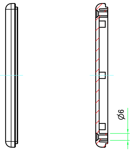
C-C ( 1 : 2 )
